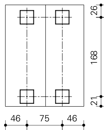
Bovenaanzicht
