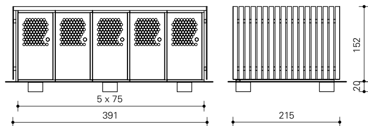
Fietskluisen
