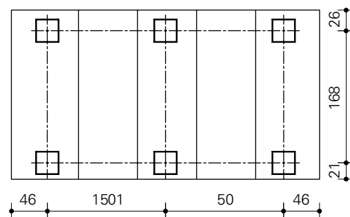
Bovenaanzicht
