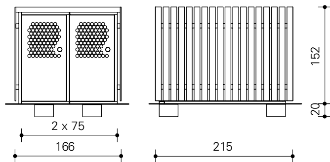
Fietskluisen
